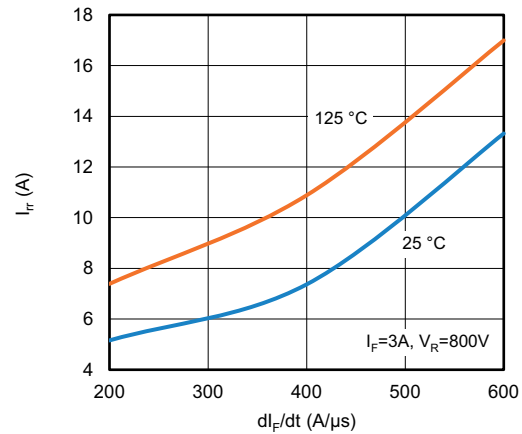
Fig. 8 - I_{rr} (A) vs. dI_F/dt
